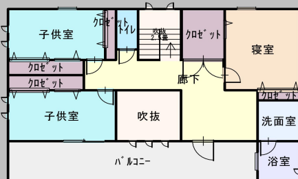
2階平面図
