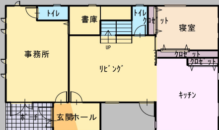
1階平面図
